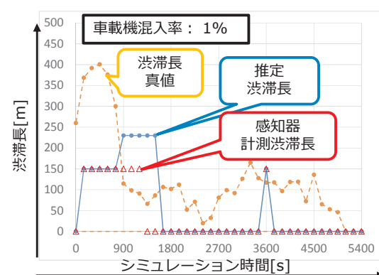
(b) 省センサー信号制御（混入率 1 %）
