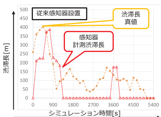
(a) 従来センサー設置
