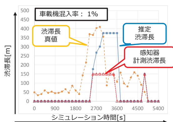
(b) 省センサー信号制御（混入率 1 %）
