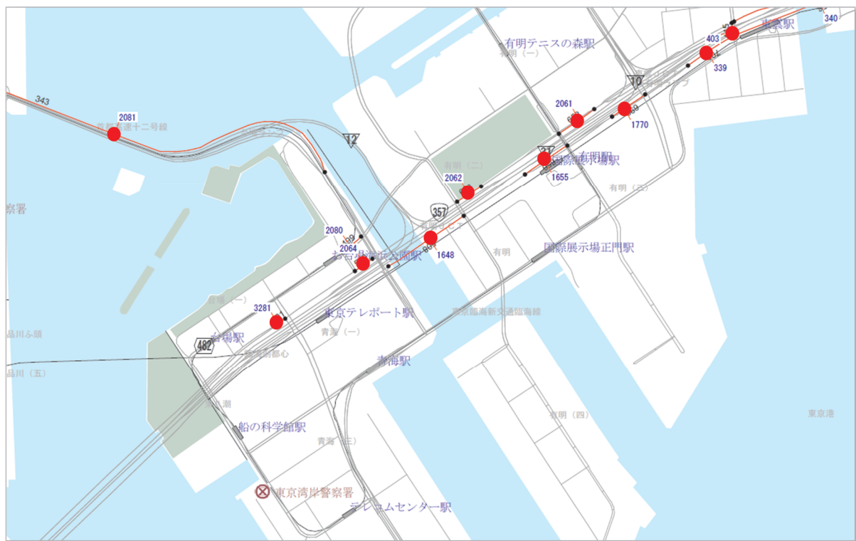
図 2.3 東京臨海部の車両感知器設置位置 ※赤丸箇所
