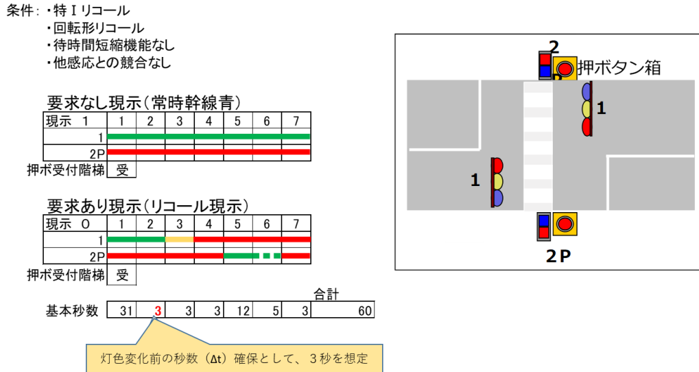
図 5.4.2 リコール 1 検証信号現示
