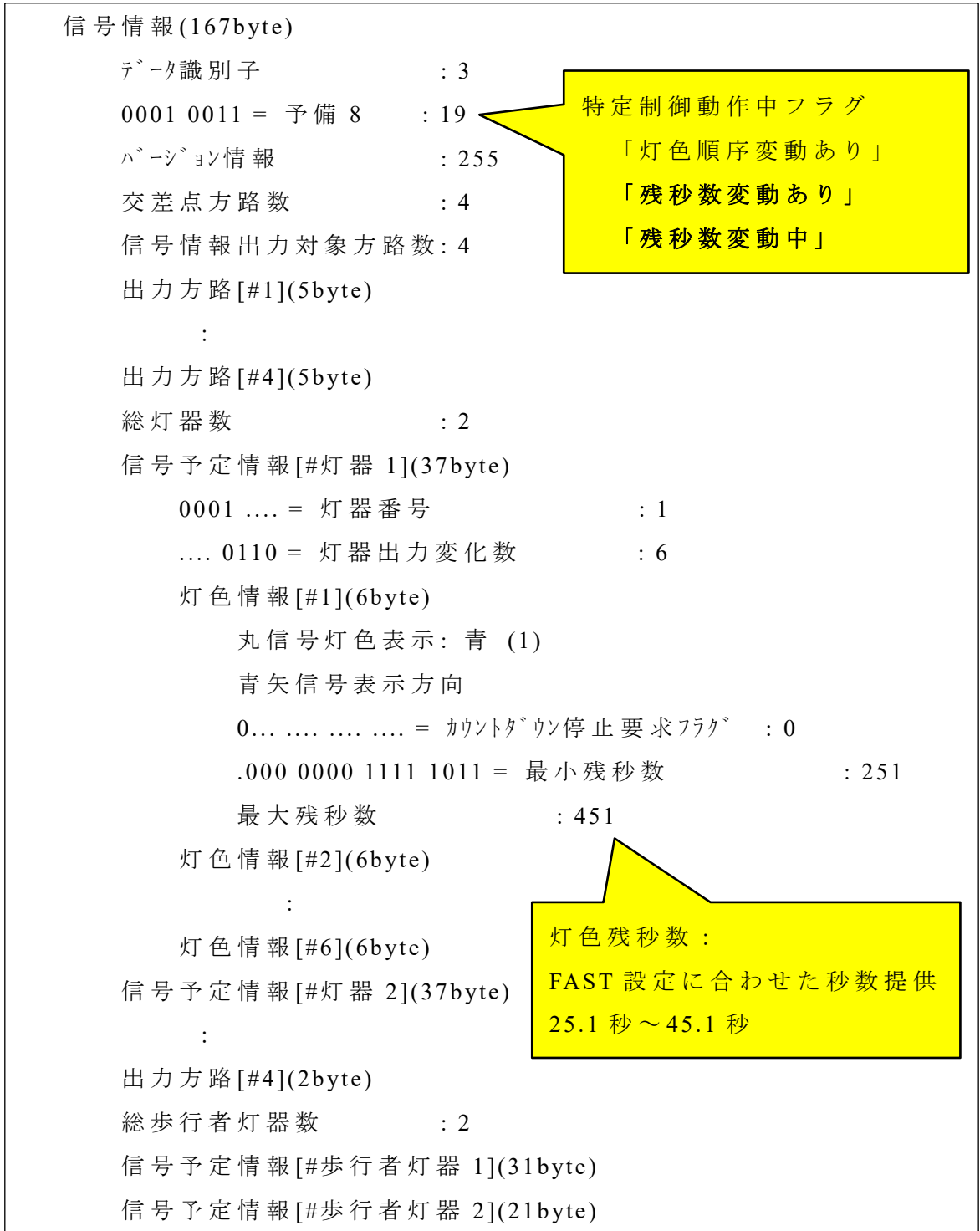
図 5.4.10 FAST 感応（短縮動作）信号情報
