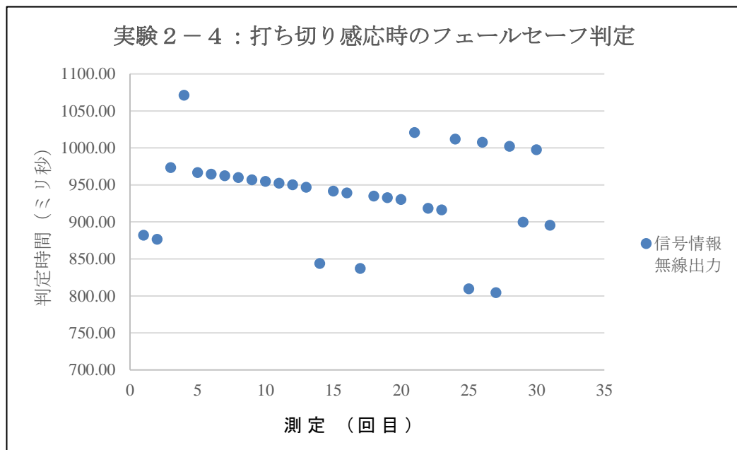
図 3.8.10 実験 2 - 4 測定結果
