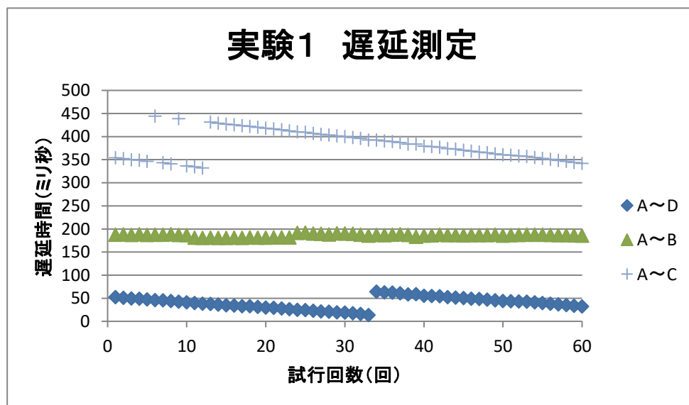
図 3.8.1 実験1測定結果
