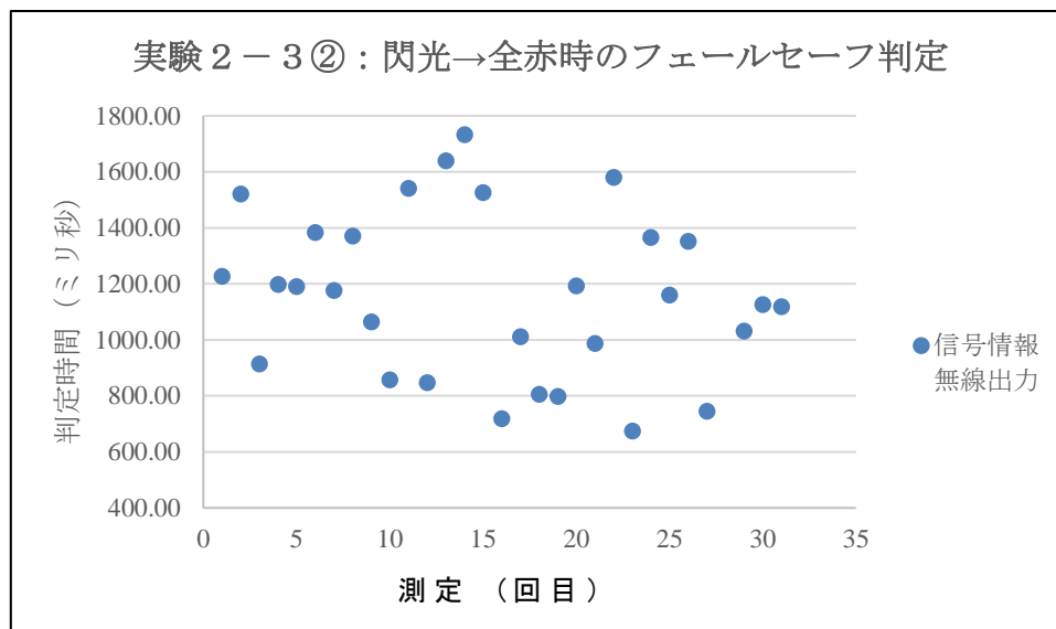
図 3.8.8 実験 2-3 ② 測定結果
