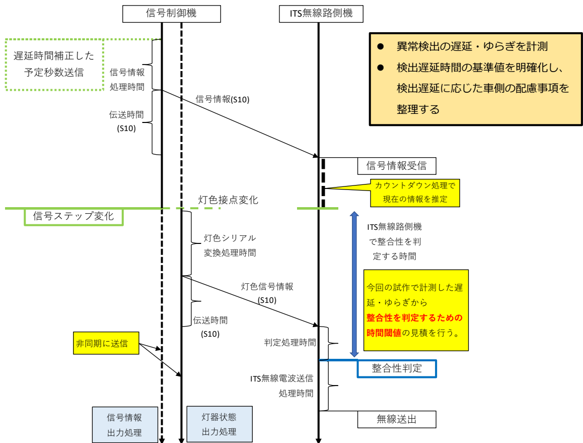
図 3.7.3 フェールセーフ機能の処理シーケンス
