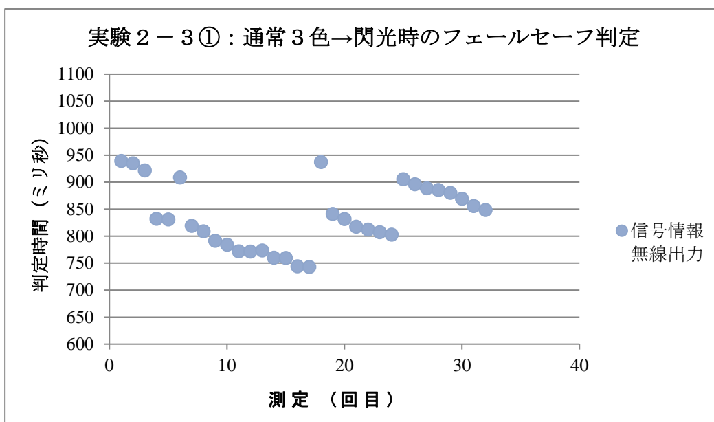
図 3.8.7 実験 2 - 3 ① 測定結果
