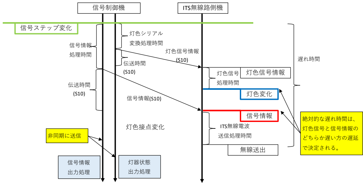
図 3.8.2 実験 1 のまとめ
