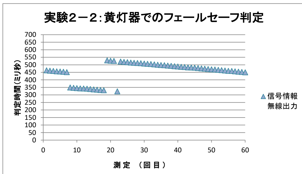
図 3.8.6 実験 2 - 2 測定結果
