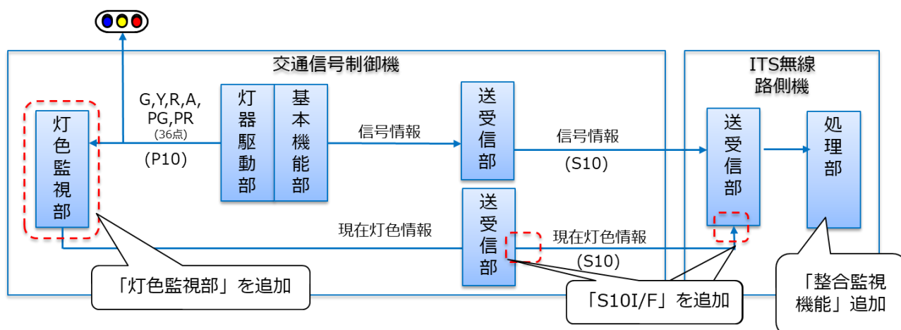
図 3.3.1 フェールセーフ機能の概要
