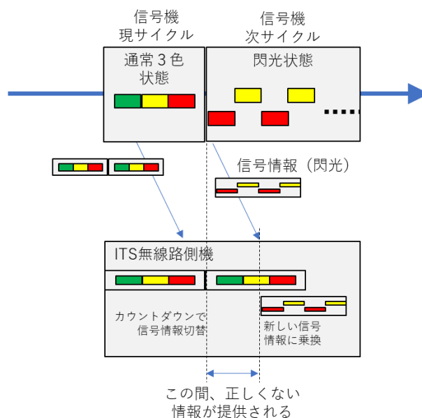
図 6.4.2 信号現示切り替わり時の信号情報
