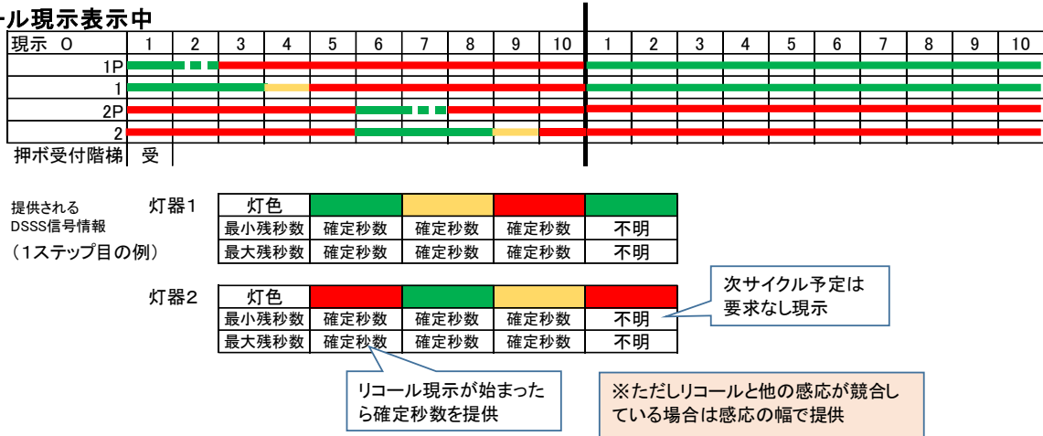
図 5.2.4 リコール制御実行中
