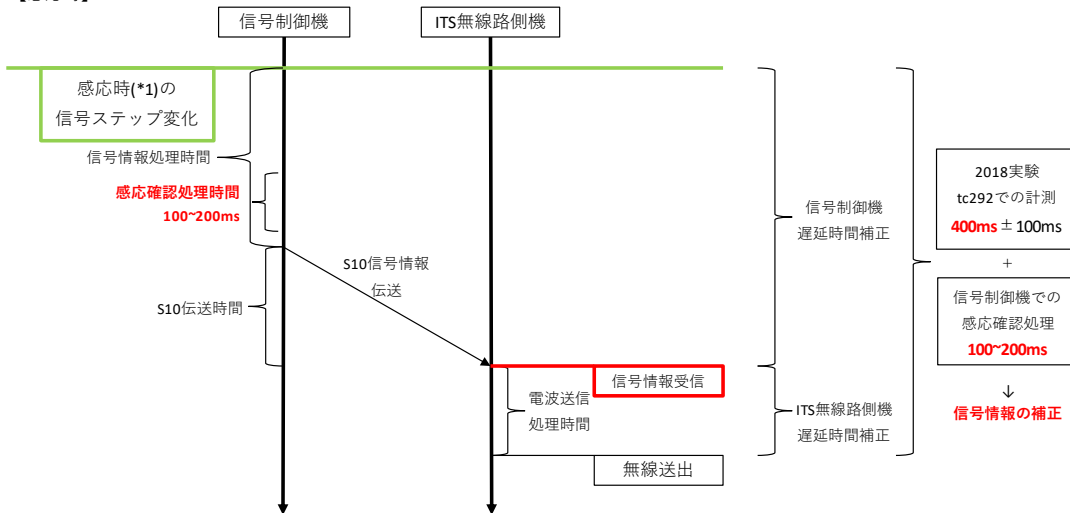
図 6.4.1 感応制御時の信号情報提供について
