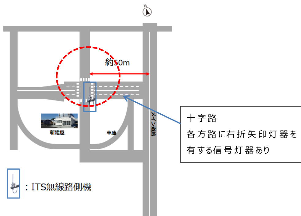
図 6.1.1 実験環境概観①
