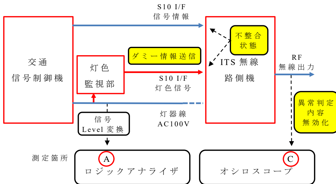
図 3.8.3 実験2の測定箇所
