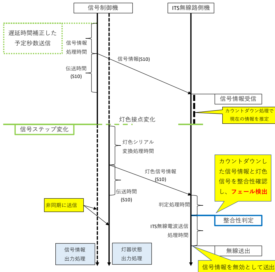
図 3.8.4 実験 2 のシーケンス
