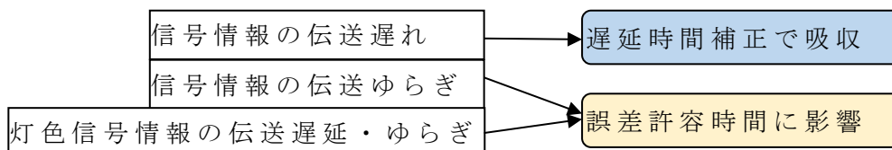
図 3.7.4 遅れ・ゆらぎの影響
