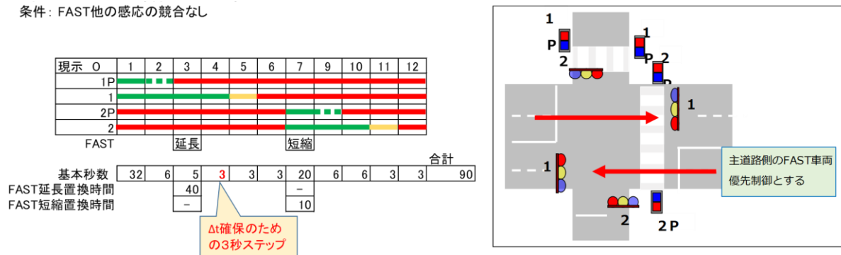
図 5.4.6 FAST 制御検証信号現示
