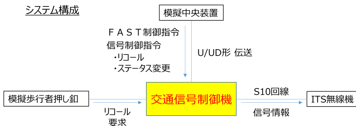
図 5.4.1 二次試作実験システム構成
