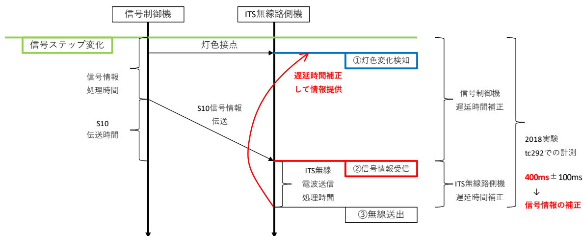
図 3.7.2 信号情報出力シーケンス
