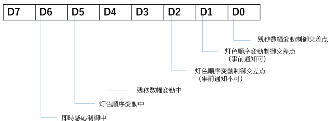
図 6.6.1 特定制御動作中フラグ定義変更案
