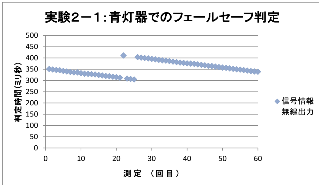
図 3.8.5 実験 2 - 1 測定結果
